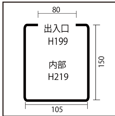
エレベーター寸法
